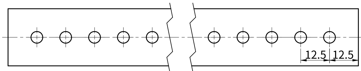
25面图样
